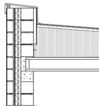
Sutapdinto stogo su keramzitu įrengimas
