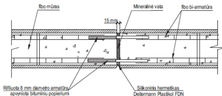
Deformacinė siūlė fibo mūre
