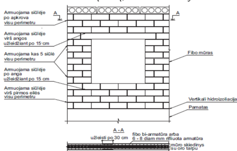
Bi - armatūros armavimas fibo 200, 250 mm mūre
