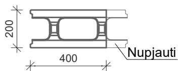
Eilinis nupjautas blokelis išorės kampui
