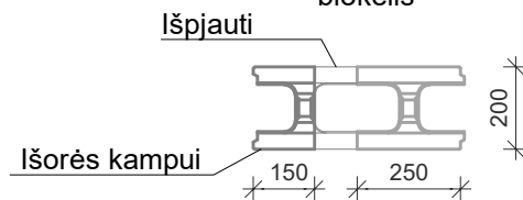
Eilinis nupjautas blokelis
