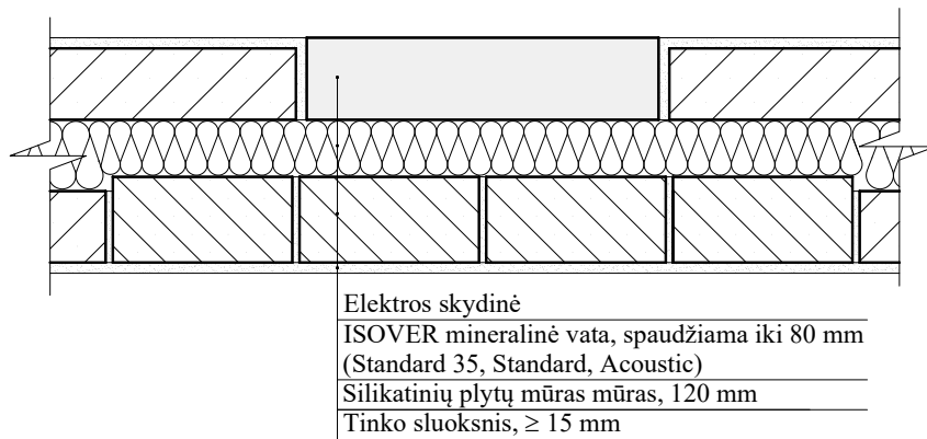
1 pav. Apskaitos prietaisų skydinės įrengimas, dalį prieš ją esančio sluoksnio mūrijant iš silikatinų plytų (horizontalus pjūvis)
